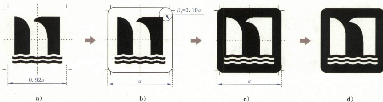
图 B.4 无边框的正方形图形标志设计示意
