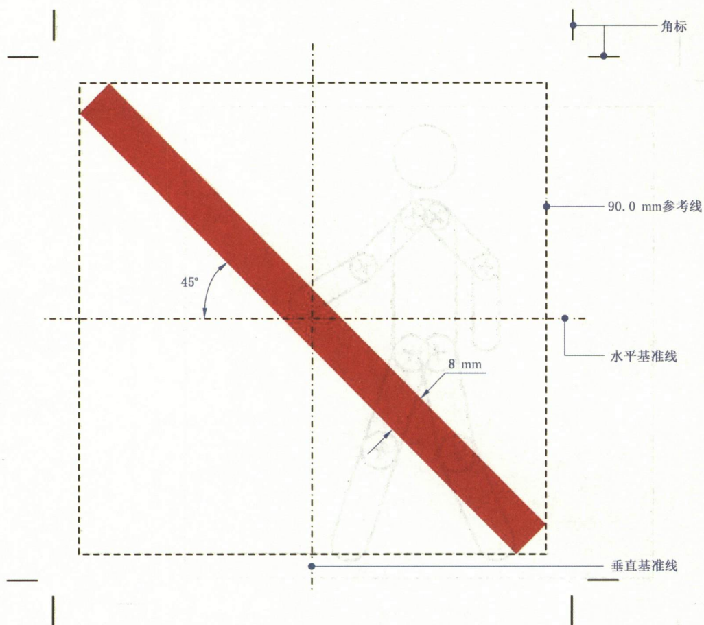
否定斜杠:穿过两条基准线的交点,与水平基准线的夹角为 45^\circ ,两端与90 mm的参考线相接,宽度为8 mm。
