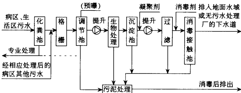
图 4.0.4-4 深度处理工艺流程
