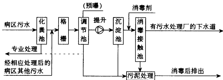
图 4.0.4-2 一级处理工艺流程(提升式)
