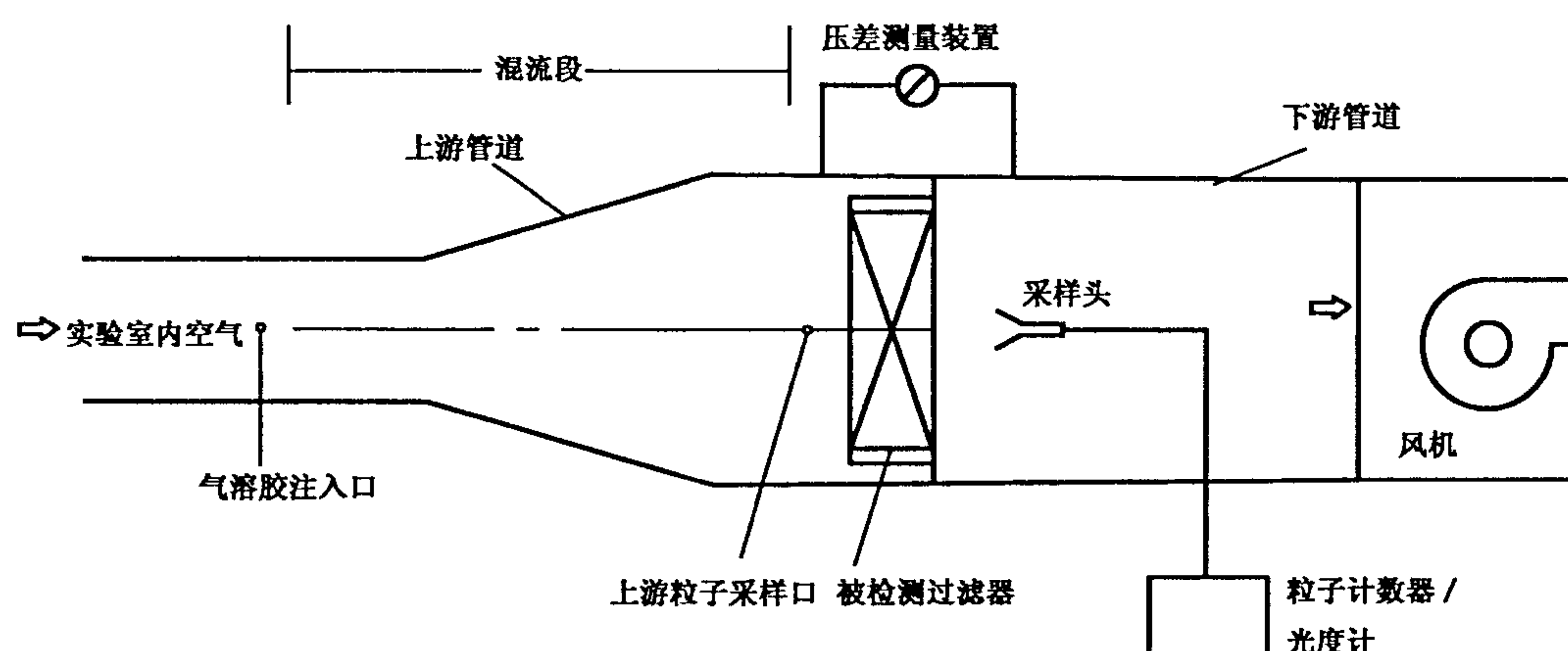
图 A.1 扫描检漏法检测示意图
