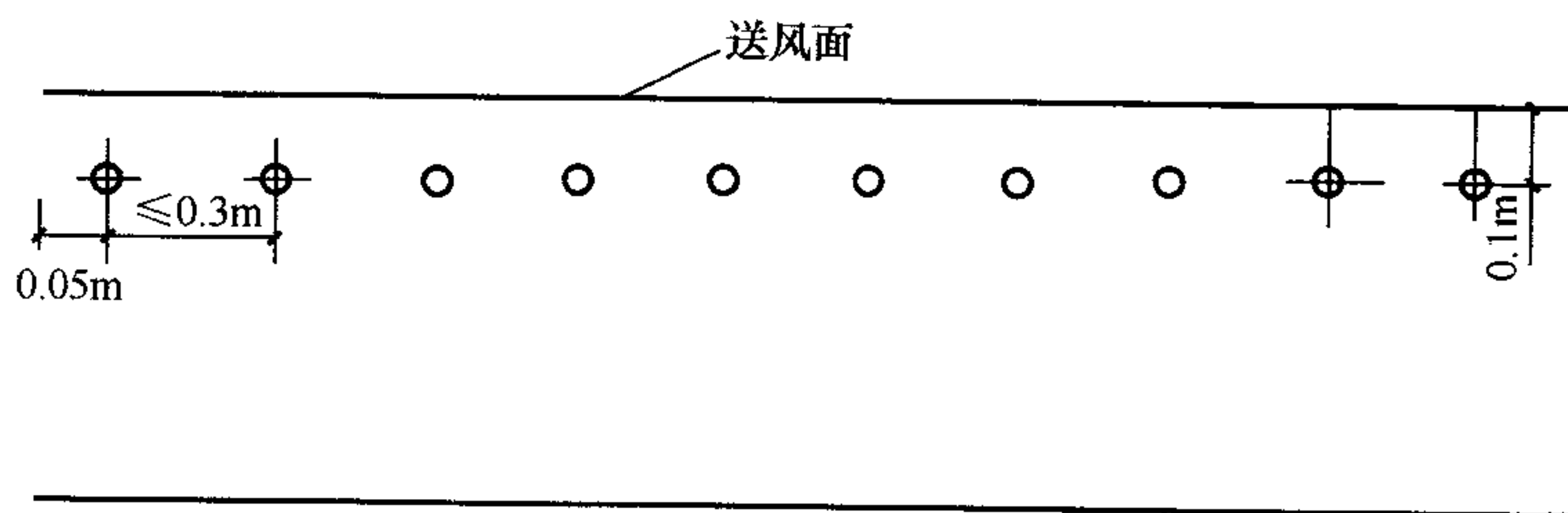
图 13.3.7 送风面速度测点断面布置
