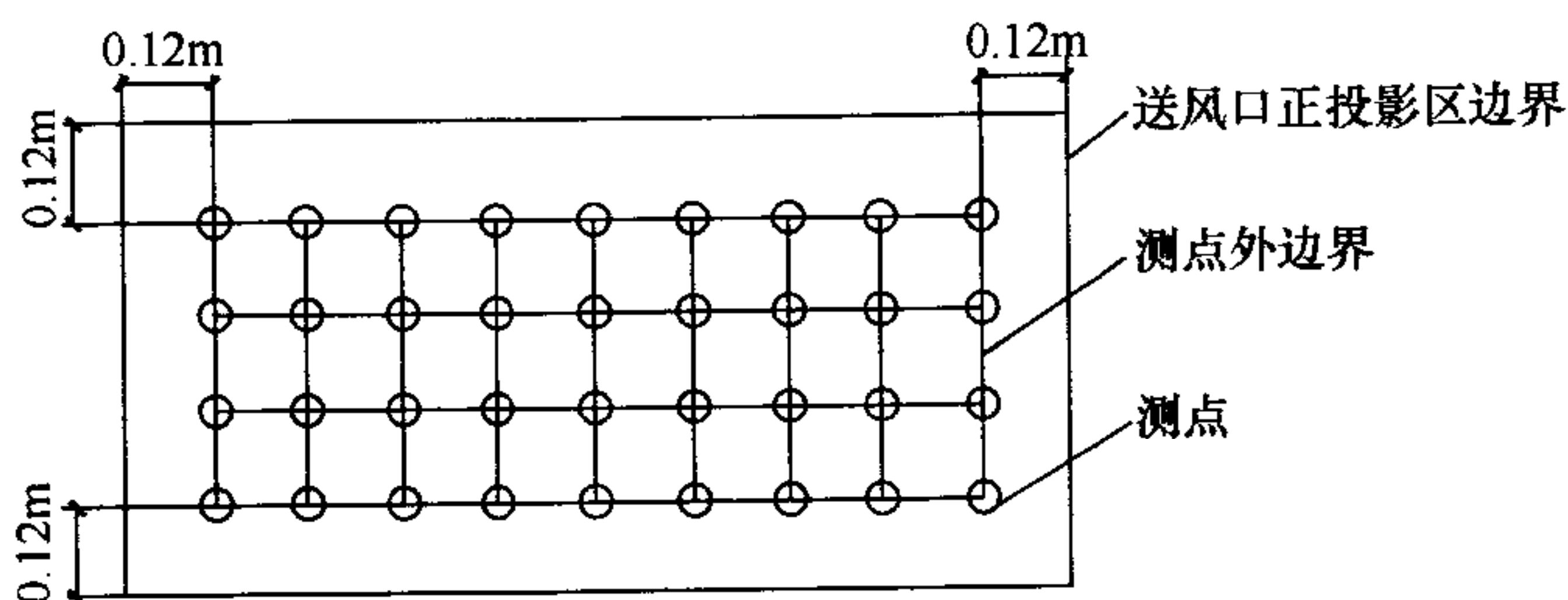
图 13.3.6 地面上 1.2m 截面风速测点平面布置
