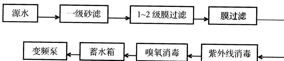
图 6.5.3 管道直饮水水处理工艺流程
