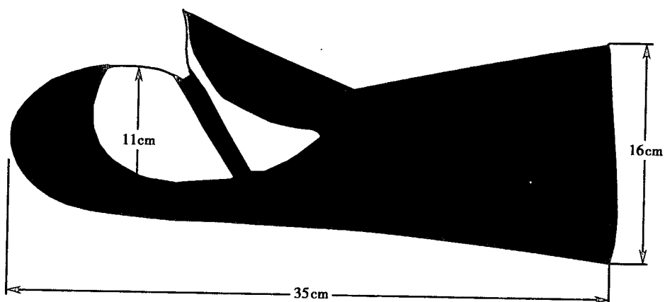
图2 连指防护手套的内部最小尺寸
